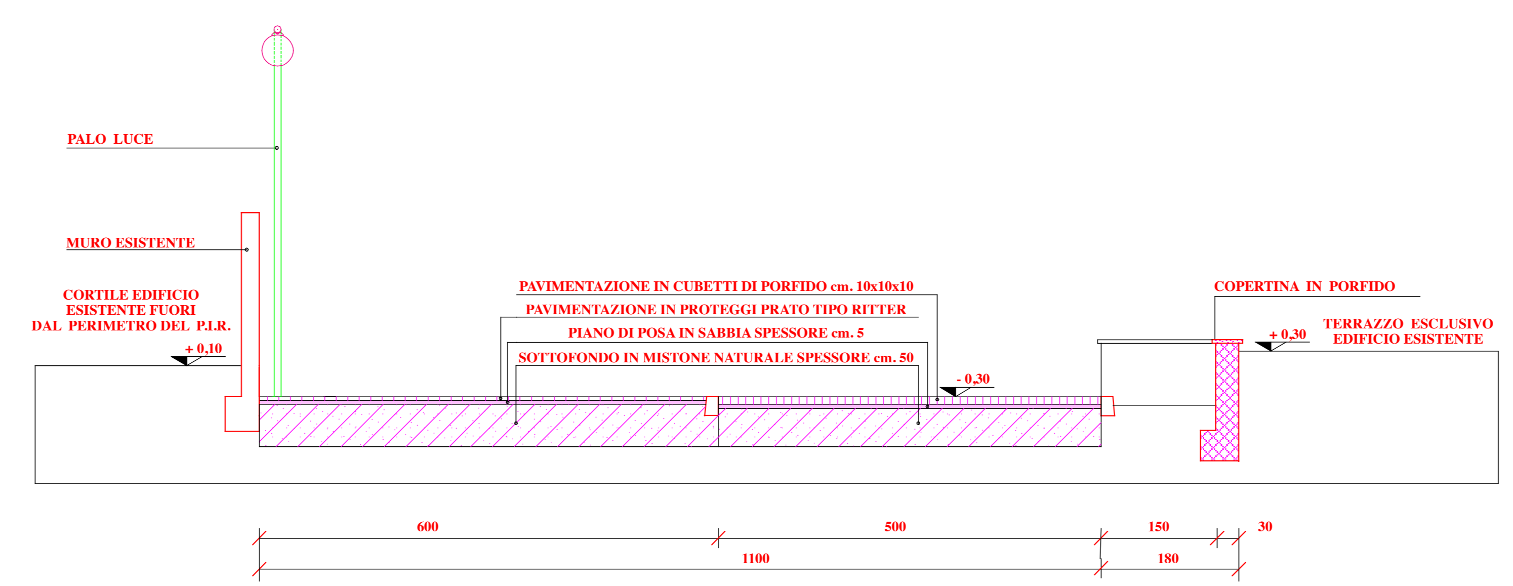
SEZIONE X-X scala 1/50
